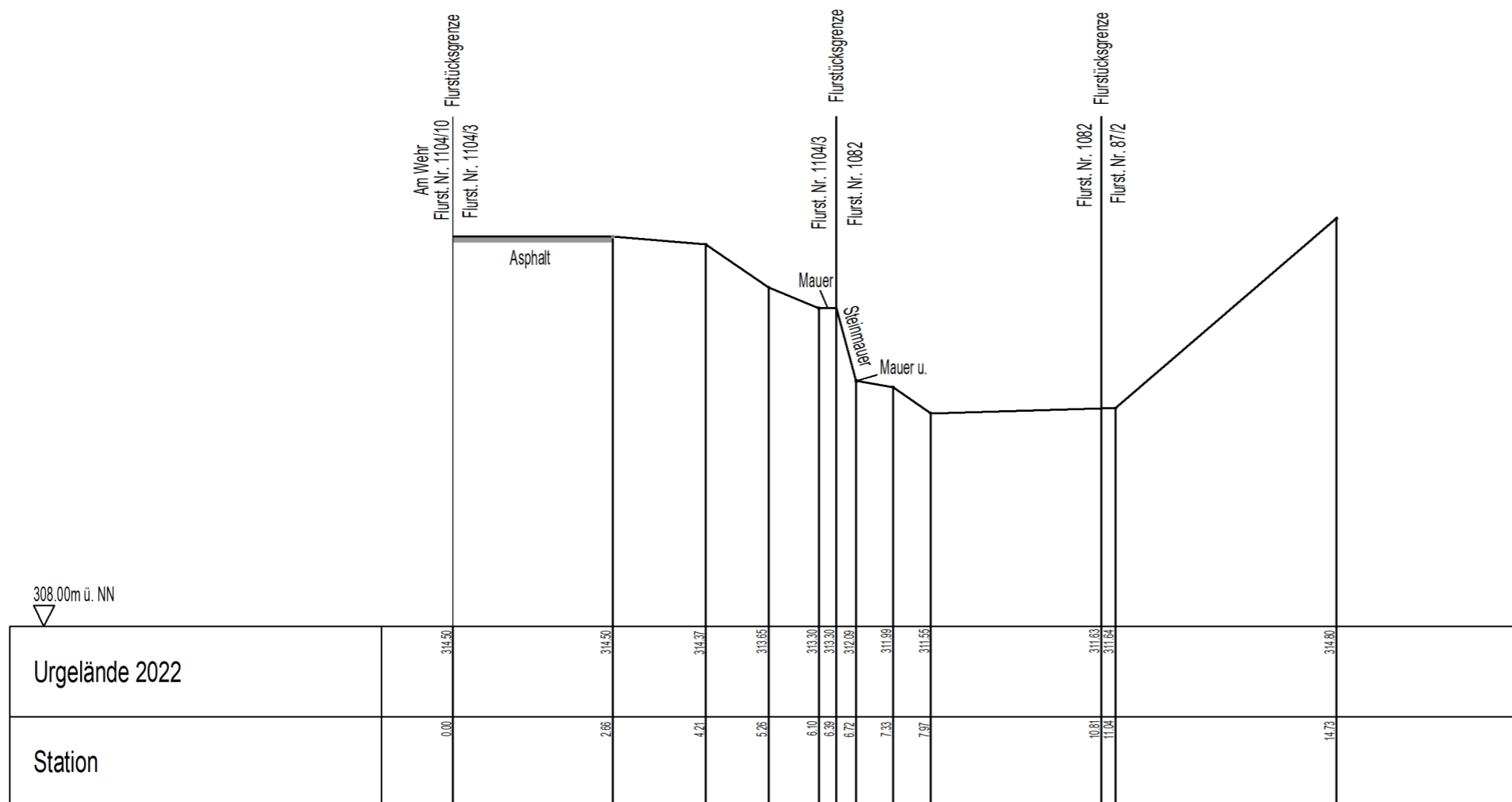
Schnitt 4
