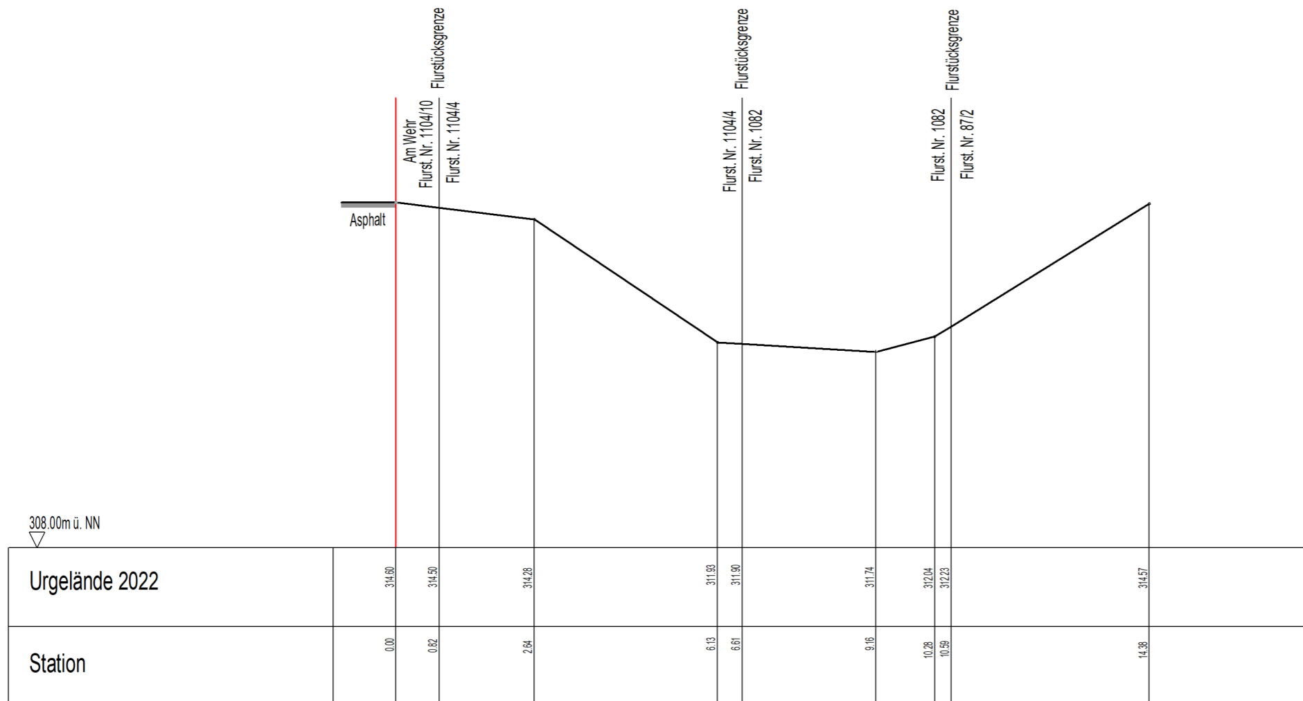
Schnitt 3
